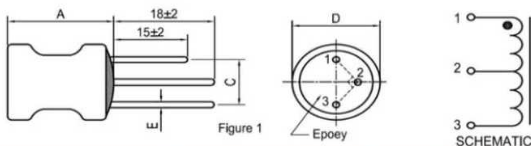
LGB3W系列三脚升压工字型电感器 图示和尺寸：（单位mm）
